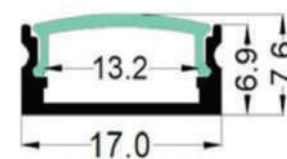
פרופיל שקוע שחור / לבן / ניקל
