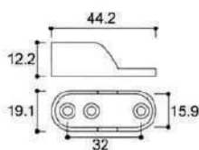
אוזן תלייה
