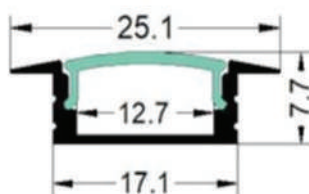
פרופיל עם שפה שחור / כבן / ניקל
