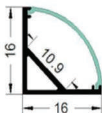
פרופיל פינה שחור / כבן / ניקל
