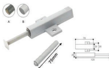
חגגון טאצ' עם בית
