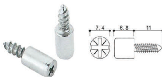
מחזיק מדף בורג ניקל
